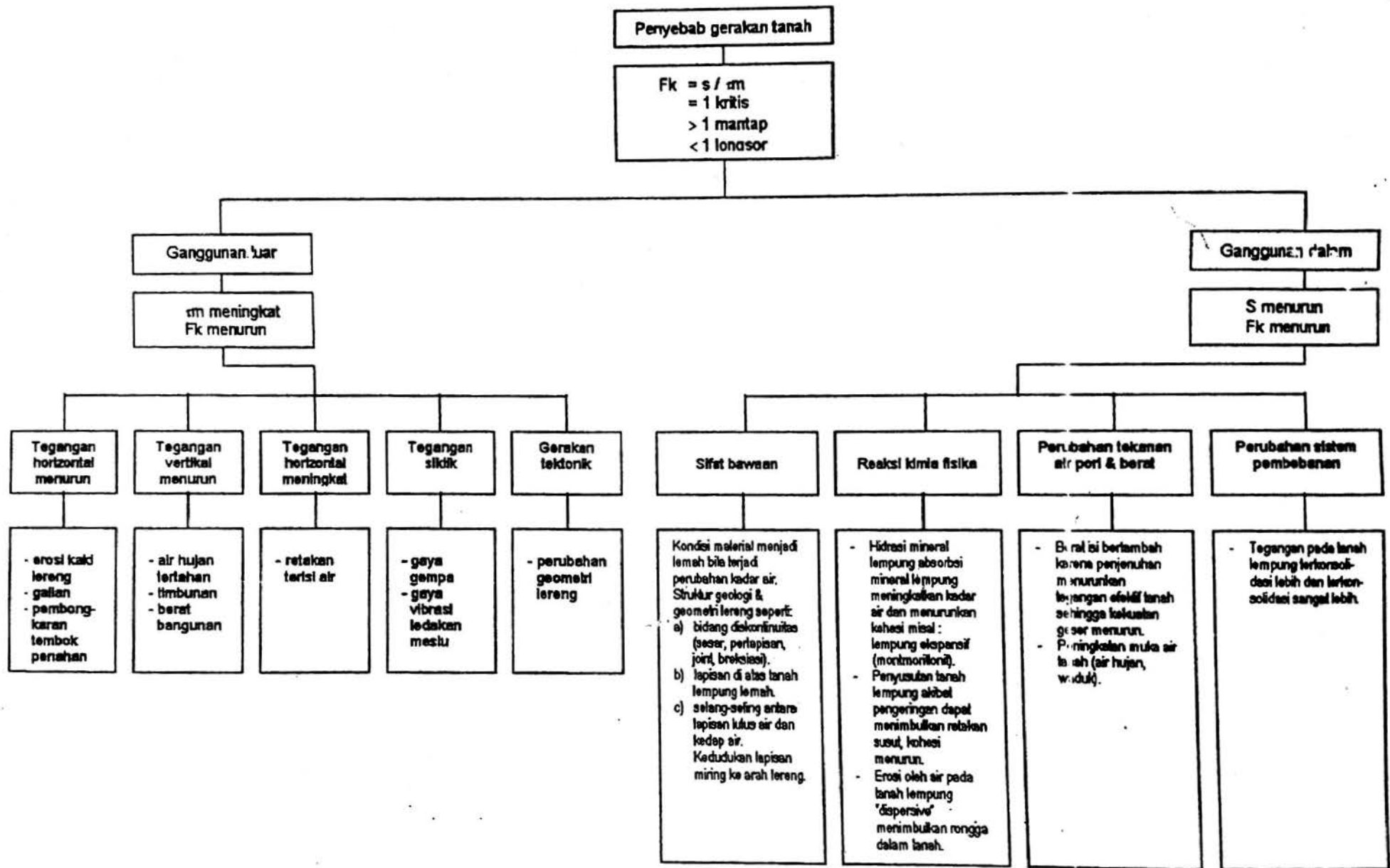
BAGAN PENYEBAB GERAKAN TANAH DITINJAU DARI KONSEPSI FAKTOR KEAMANAN
