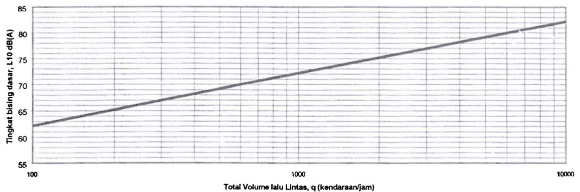
Grafik 1 Prediksi tingkat bising dasar, L_{10} 1 jam
