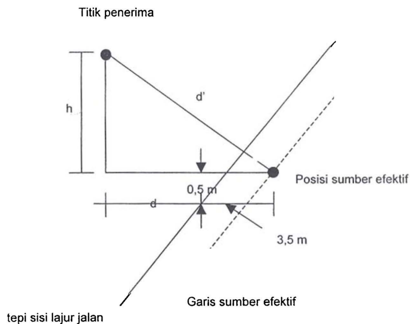
Gambar 2 Skema jarak titik penerima dan sumber bunyi
