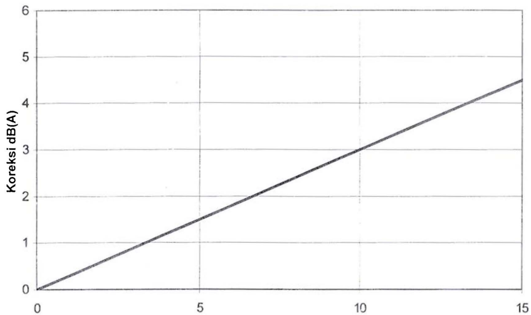
Grafik 4 Faktor koreksi gradien
