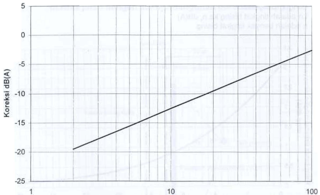
Grafik 8 Koreksi sudut pandang jalan (θ)
