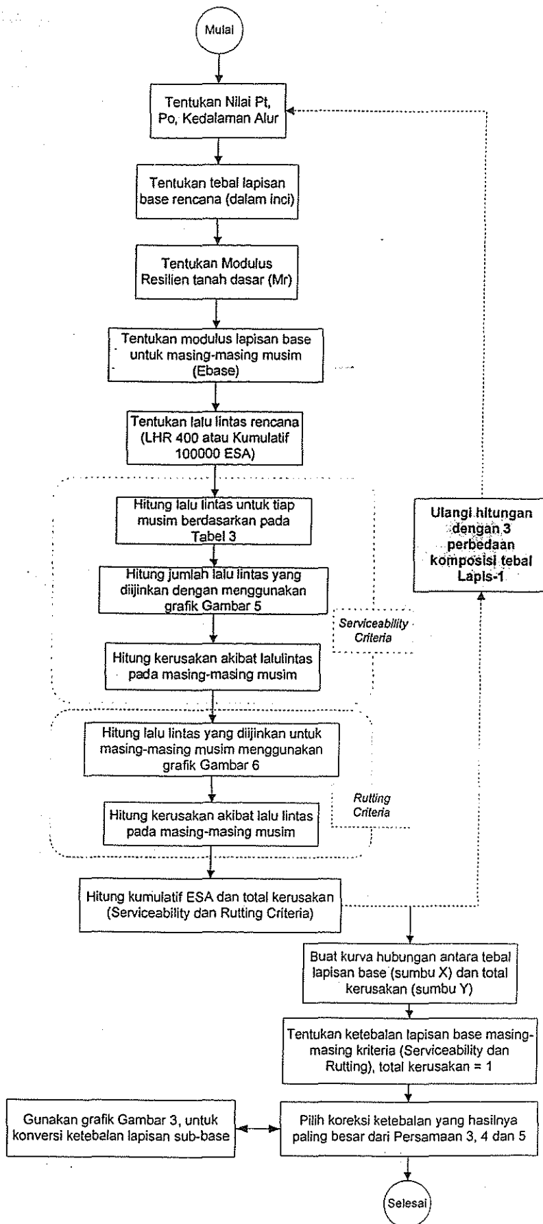
Gambar 4 - Diagram alir langkah perencanaan tebal jalan kerikil
