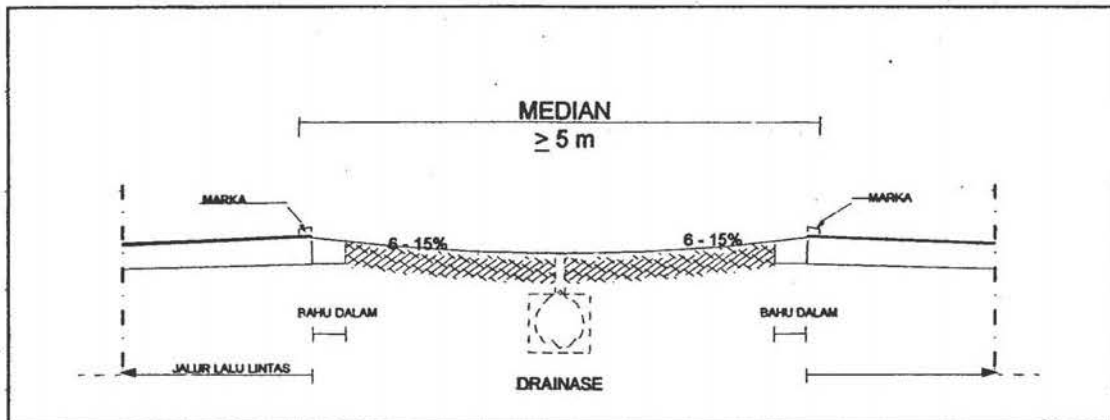
Gambar 6 Median yang diturunkan
