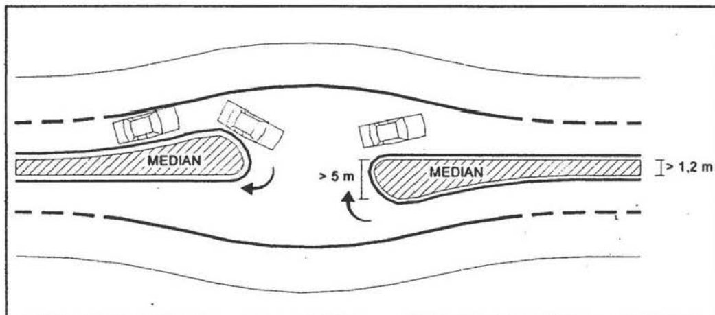
Gambar 7 Median pada daerah pendekat bukaan
