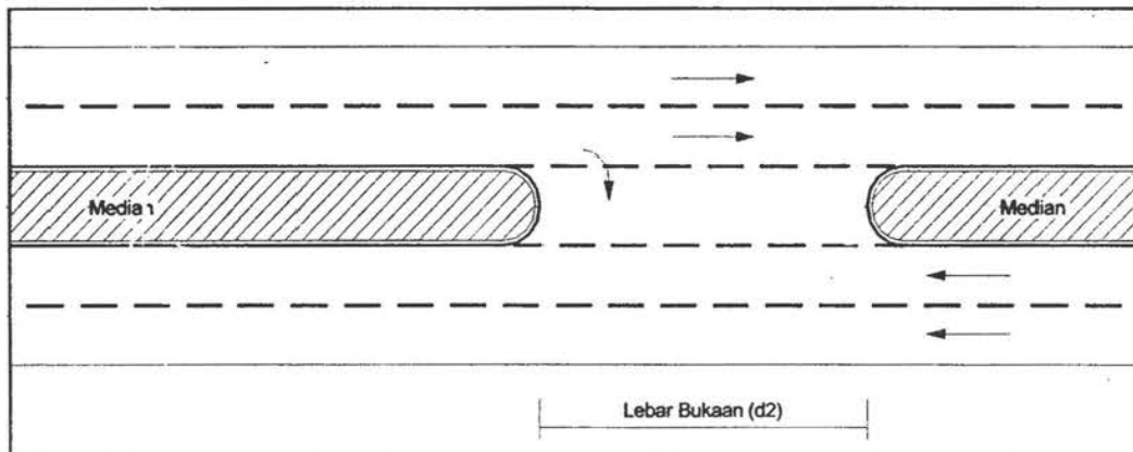
Gambar 9 Lajur tunggu pada bukaan
