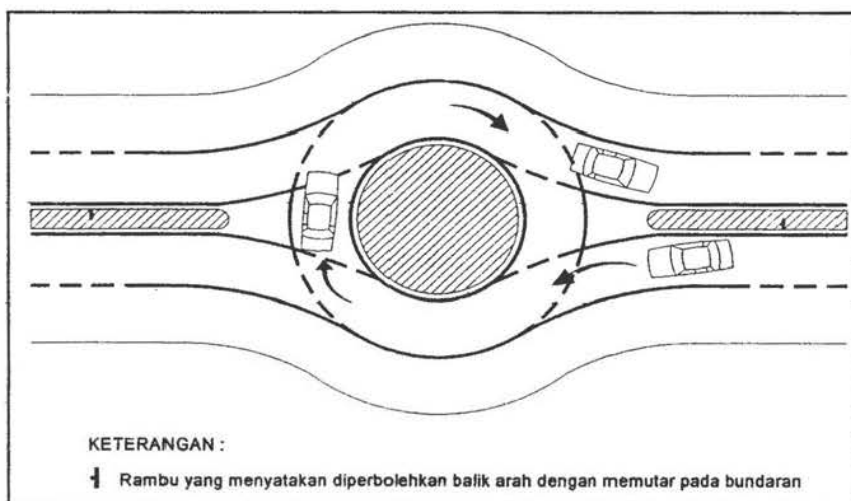
Gambar A-3 Bukaan median dengan bentuk bundaran
