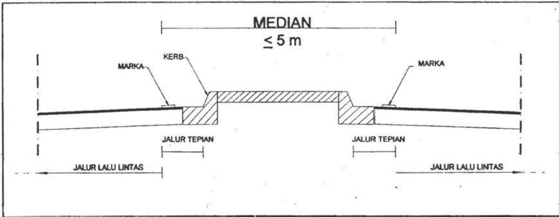
Gambar 3 Median yang ditinggikan
