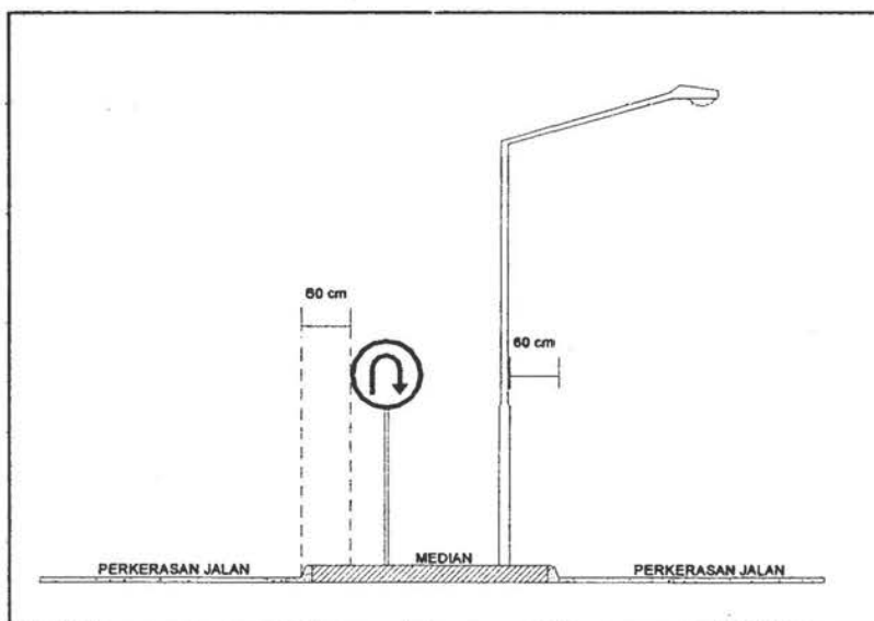
Gambar 11 Lebar ruang bebas kendaraan
