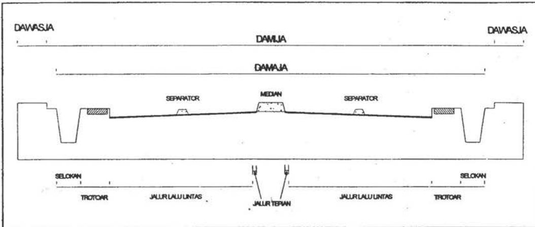
Gambar 1 Potongan melintang jalan
