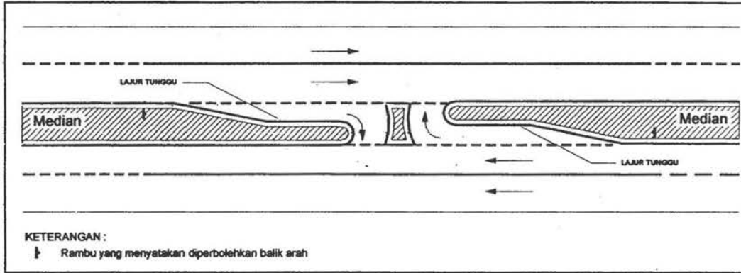
Gambar A-1 Median dilengkapi lajur tunggu
