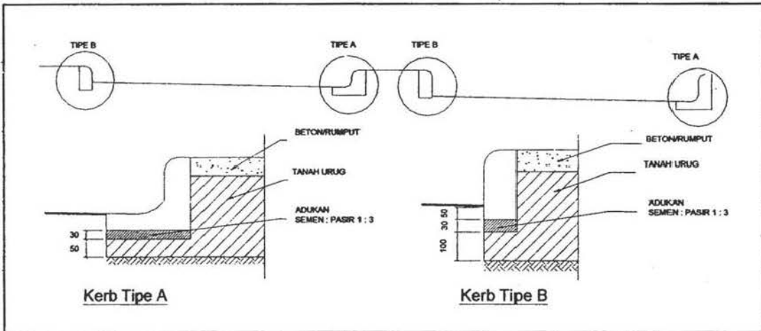
Gambar 4 Sisi luar median yang dilengkapi kereb
