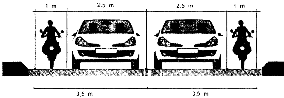
Gambar 4 - Potongan melintang lebar lajur minimum
