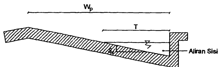
Gambar 4 – Saluran tepi
