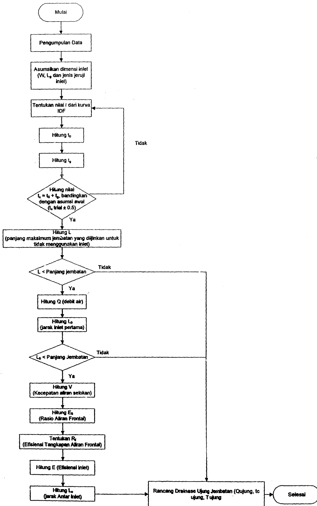
Gambar 6 - Diagram alir perancangan inlet jembatan
