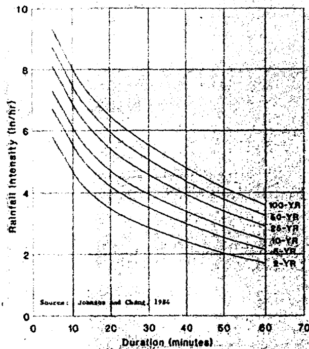
Gambar A.1-Kurva Intensitas Durasi Frekuensi (IDF)
