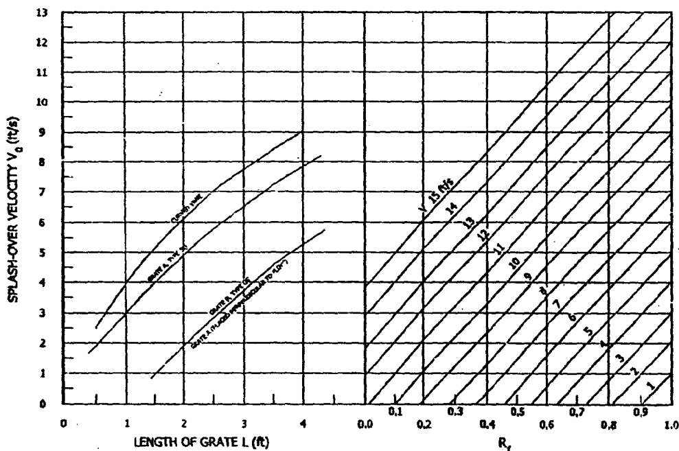
Gambar 5 - Efisiensi tangkapan aliran frontal untuk berbagai jenis Jeruji (HEC 12)
