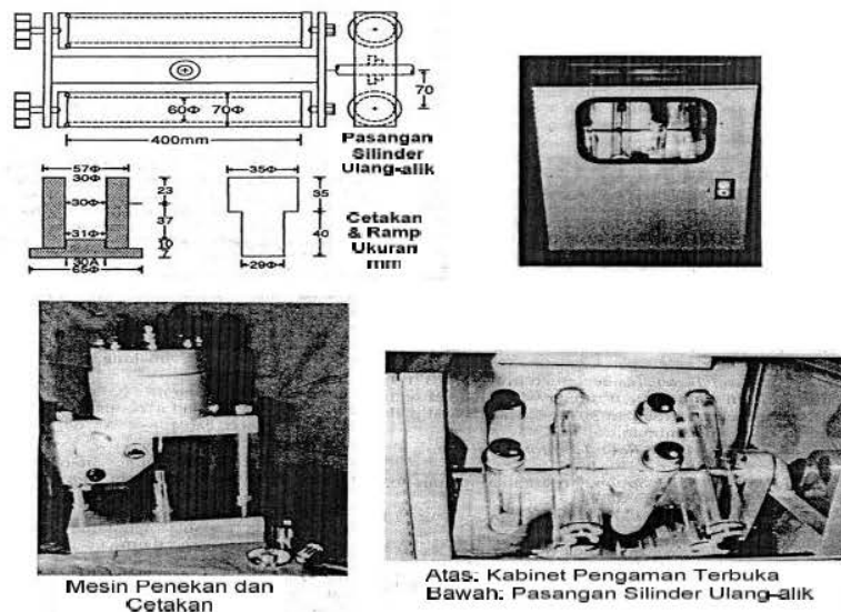
Gambar E.1 - Mesin abrasi Sculze-Breuer
