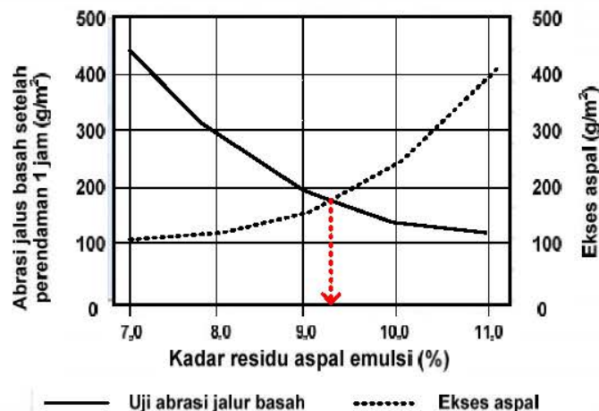
Gambar F.3 - Kadar residu aspal emulsi optimum lapis permukaan mikro
