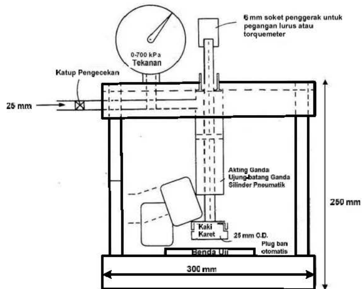
Gambar B.1 - Alat uji kohesi (tampak depan)
