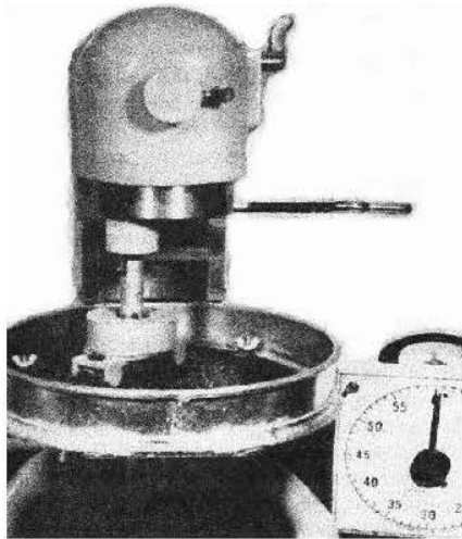
Gambar C.1 - Benda uji dalam piring slap untuk diuji (gambaran alat C-100)
