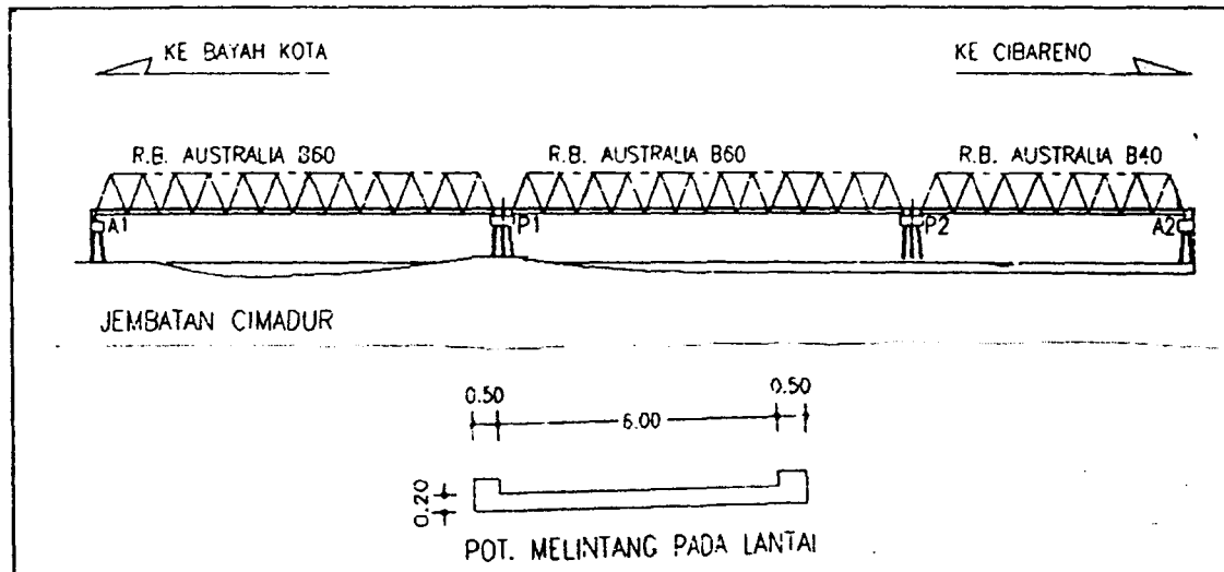
Gambar 7. Bangunan Atas Jembatan Cimadur
