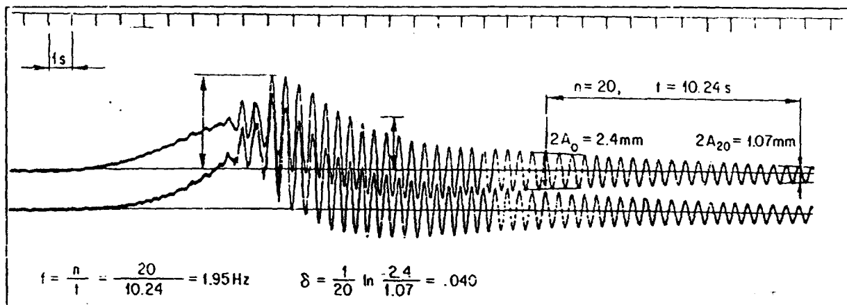
Gambar 6 : Interpretasi rekaman getaran tipikal
