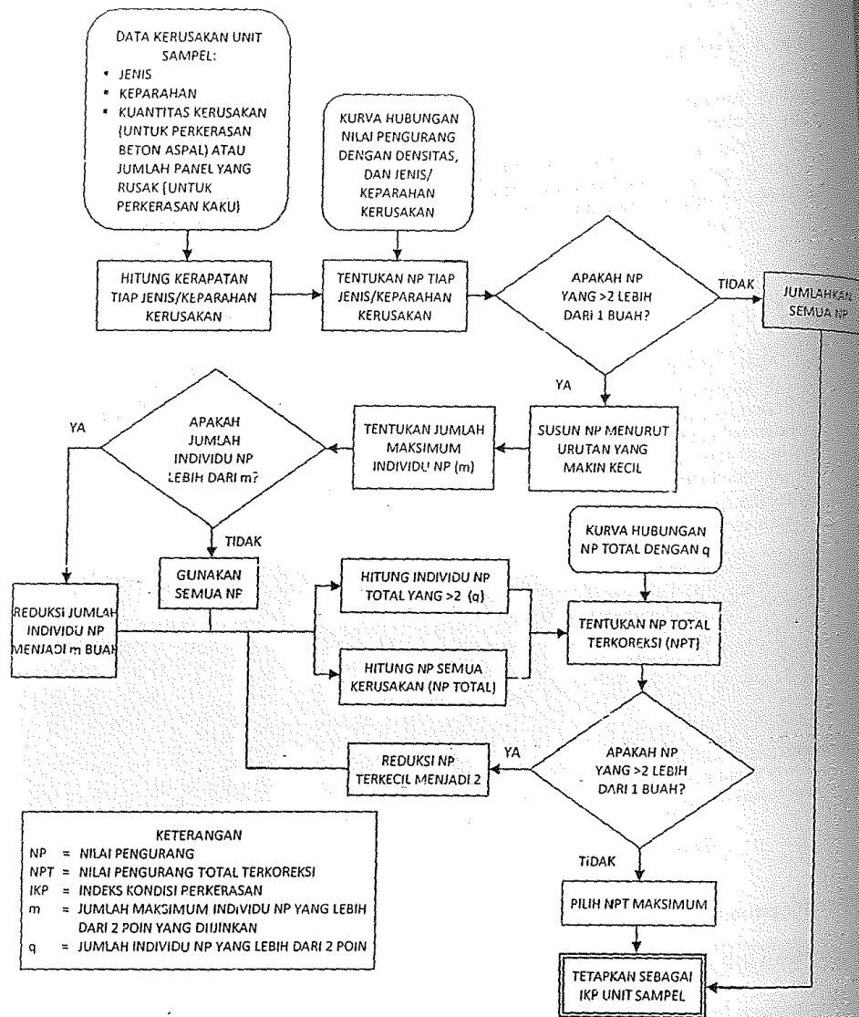
Gambar 44 - Tahapan penentuan IKP unit sampel
