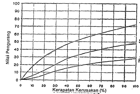
I - Tambalan besar, tambalan galian utilitas
