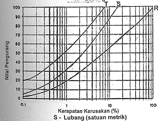
Gambar 45 - Grafik nilai pengurang (NP) perkerasan beraspal (lanjutan)
