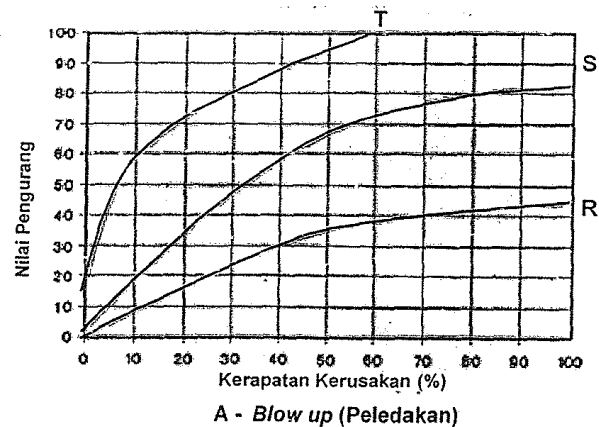
Gambar 48 - Grafik nilai pengurang (NP) perkerasan kaku
