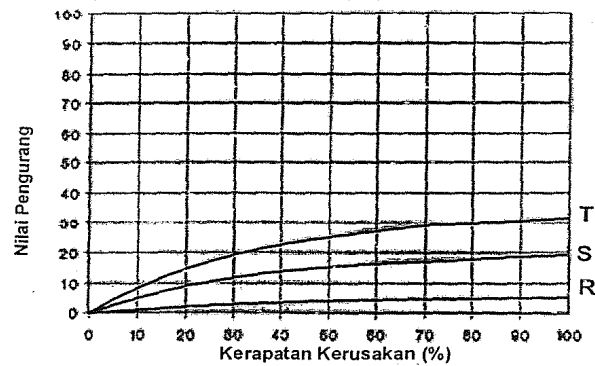
G - Penanggaan lajur/bahu
