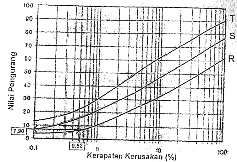
Gambar C.3 - Kurva hubungan nilai pengurang dan kerapatan kerusakan retak kulit buaya
