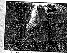
A. Retak kulit buaya keparahan rendah
