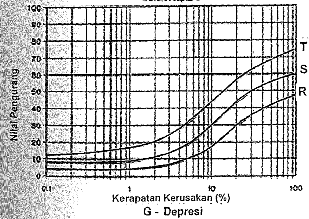
Gambar 45 - Grafik nilai pengurang (NP) perkerasan beraspal (lanjutan)
