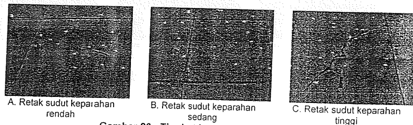
Gambar 26 - Tingkat keparahan retak sudut
