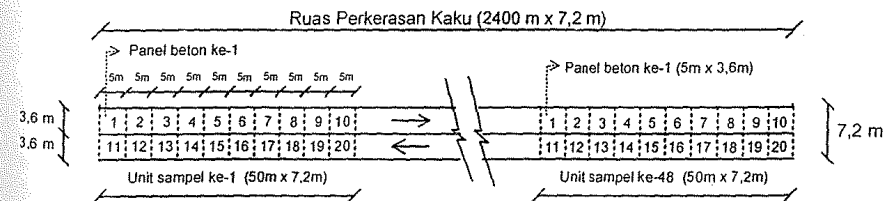
Gambar 3 - Contoh pembagian ruas perkerasan kaku menjadi unit sampel
