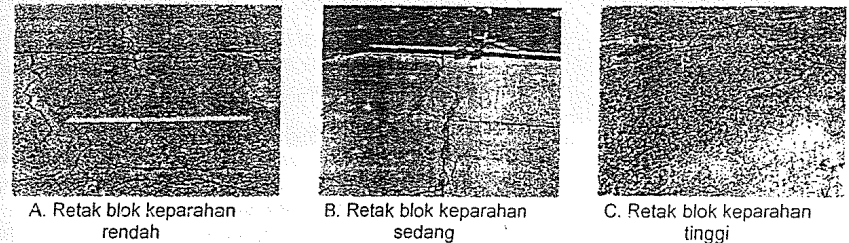
Gambar 7 - Tingkat keparahan retak blok
