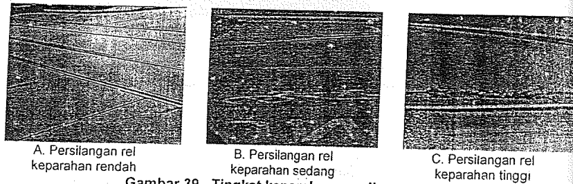
Gambar 39 - Tingkat keparahan persilangan rel
