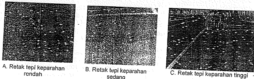
Gambar 11 - Tingkat keparahan retak tepi
