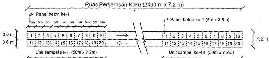
Gambar D.1 - Contoh pembagian ruas perkerasan kaku menjadi unit sampel
