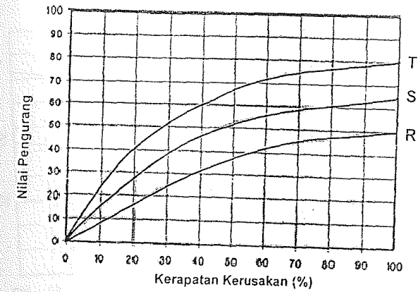
B - Retak sudut
