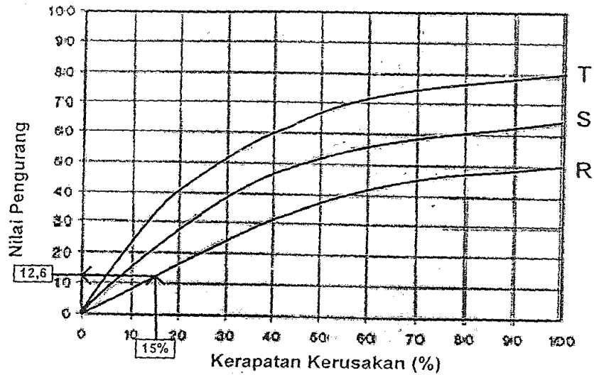
Gambar D.3 - Kurva hubungan nilai pengurang dan kerapatan retak sudut
