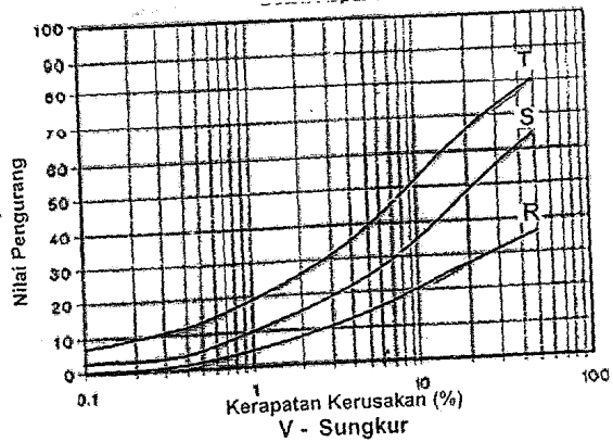
Gambar 45 - Grafik nilai pengurang (NP) perkerasan beraspal (lanjutan)
