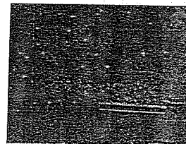
C. Retak selip keparahan tinggi
