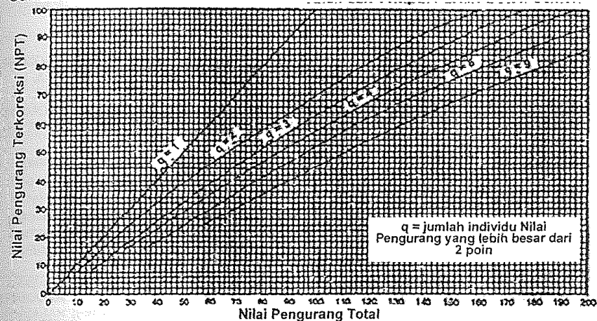
Gambar 49- Kurva menghitung nilai pengurang terkoreksi (NPT) untuk perkerasan kaku bersambung
