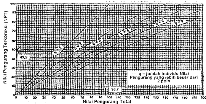
Gambar D.5 - Kurva menghitung nilai pengurang terkoreksi (NPT) untuk perkerasan kaku
