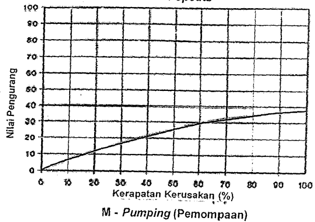
Gambar 48 - Grafik nilai pengurang (NP) perkerasan kaku (lanjutan)
