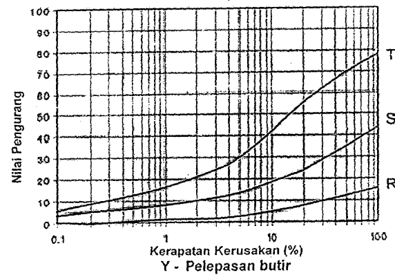
Gambar 45 - Grafik nilai pengurang (NP) perkerasan beraspal (lanjutan)
