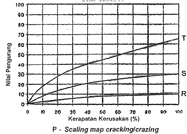
Gambar 48 - Grafik nilai pengurang (NP) perkerasan kaku (lanjutan)
