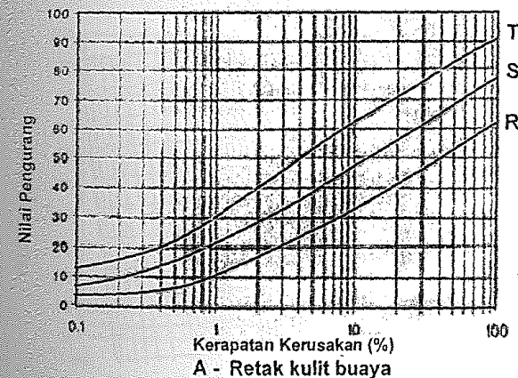
Gambar 45 - Grafik nilai pengurang (NP) perkerasan beraspal
