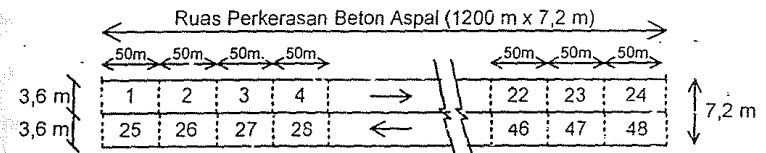
Gambar C.1 - Pembagian ruas perkerasan beton aspal menjadi unit sampel
