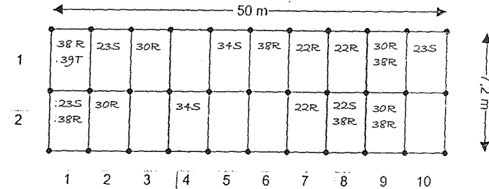
Gambar D.2 - Contoh hasil survei kerusakan perkerasan kaku pada unit sampel nomor 2
