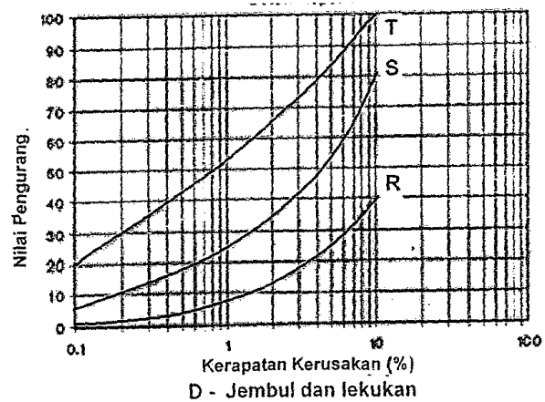
Gambar 45 - Grafik nilai pengurang (NP) perkerasan beraspal (lanjutan)
