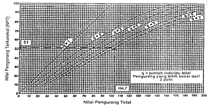
Gambar C.5 - Kurva untuk menentukan nilai pengurang terkoreksi (unit sampel perkerasan beton aspal)
