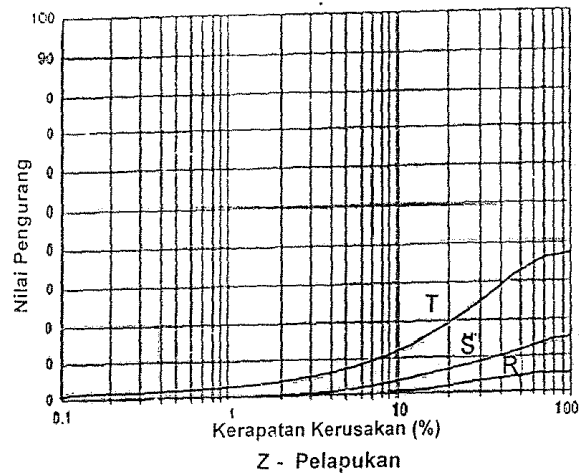
Gambar 45 - Grafik nilai pengurang (NP) perkerasan beraspal (lanjutan)
