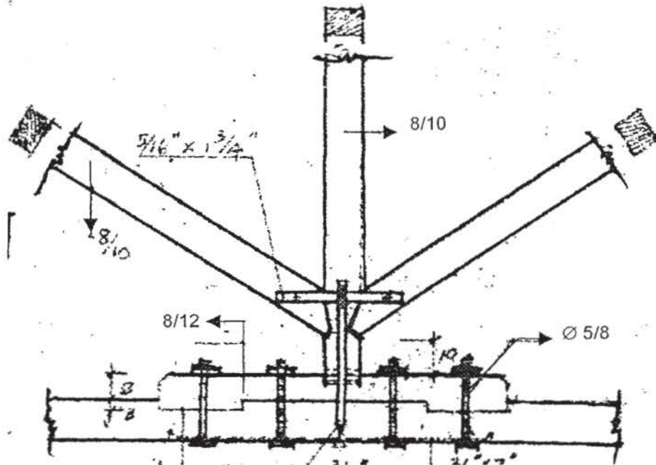
Gambar 23 Detail Sambungan pada Tumpuan Tengah
