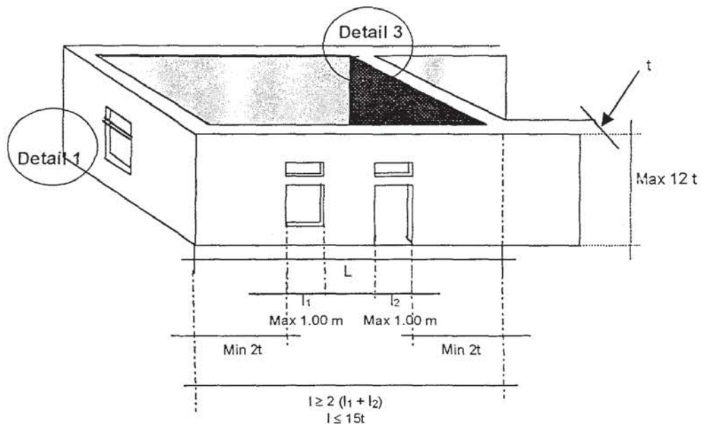
Gambar 7 Dinding dengan Masing-masing Bukaan
