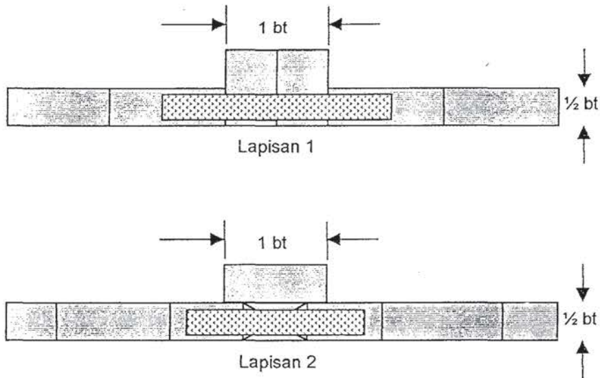
Gambar 10 Detail Sambungan atau Pertemuan Dinding Penyekat
