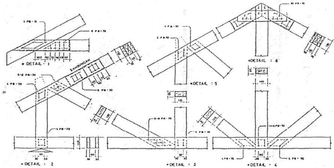
Gambar 21 Detail Sambungan Rangka Papan Paku
