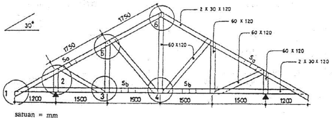
Gambar 20 Rangka Atap Kuda-kuda Kayu dan Papan Paku
