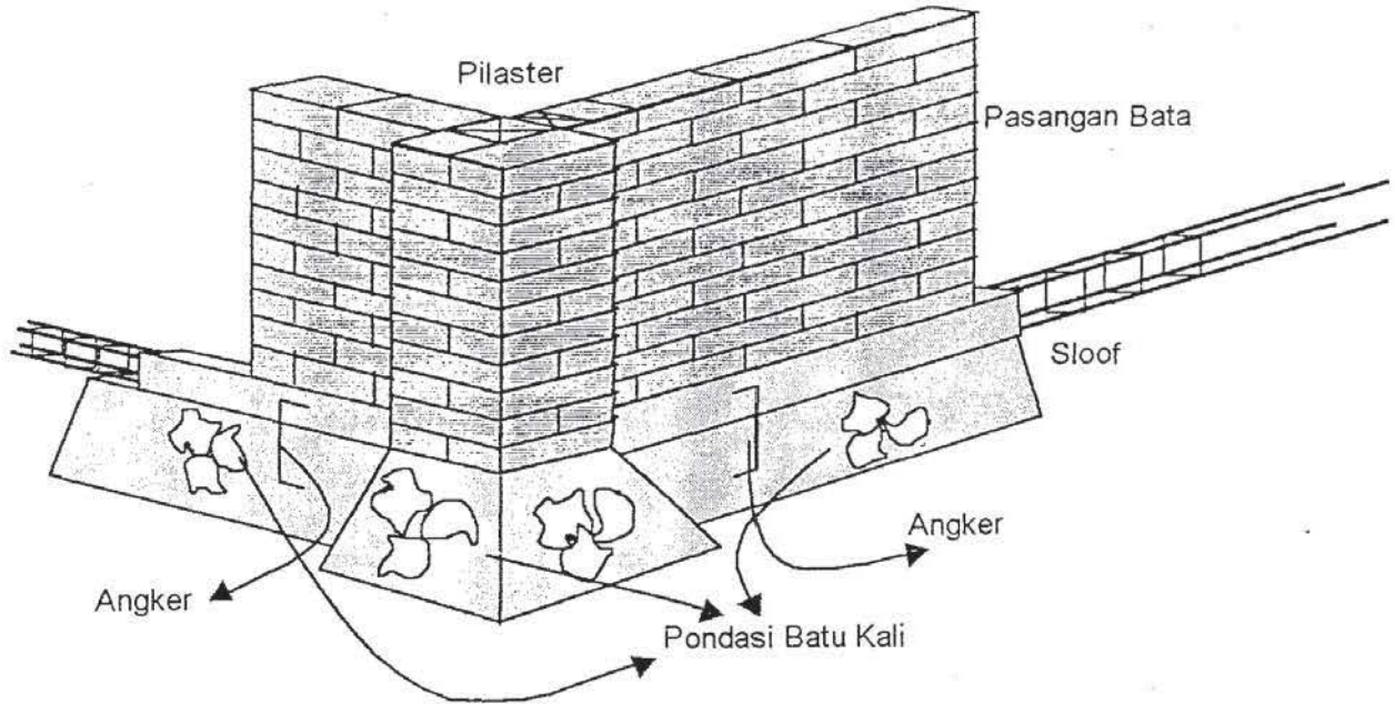
Gambar 8 Detail Sambungan atau Pertemuan
