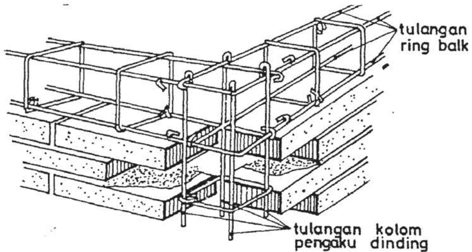
Gambar 18 Detail Penulangan Ikatan Kolom dan Ring Balok
