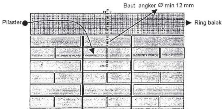
Gambar 13 Detail Pemasangan Angker antara Ring Balok dan Pilaster
