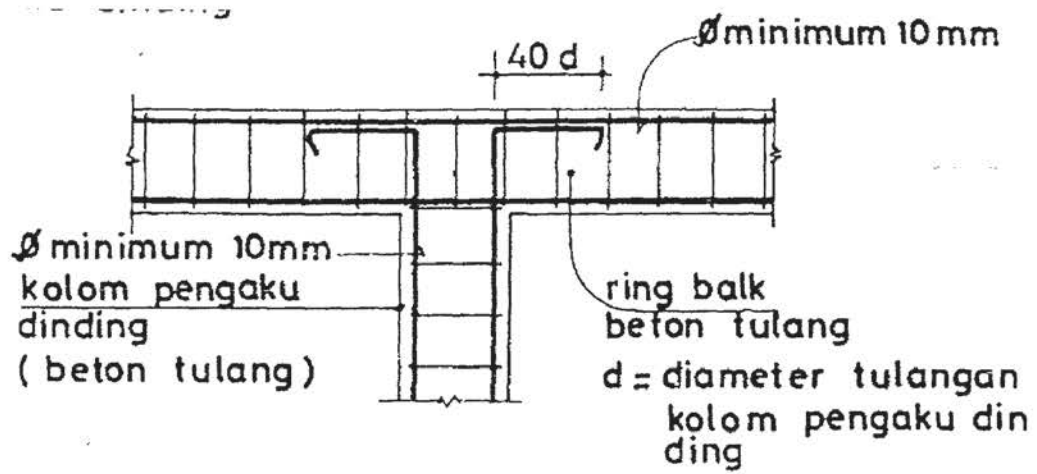
Gambar 17 Detail Penulangan Ikatan Kolom dan Ring Balok
