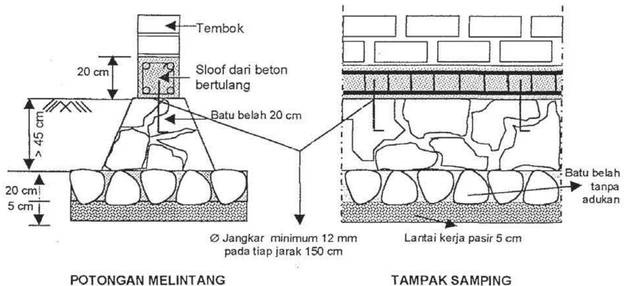
Gambar 5 Detail Pondasi Melintang dan Tampak Samping
