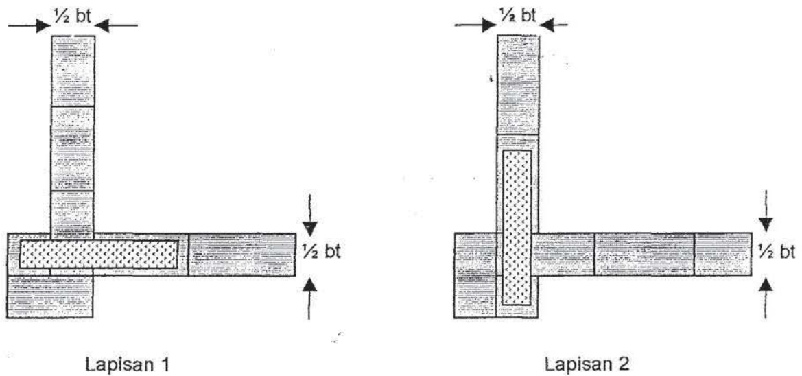
Gambar 9 Detail Sambungan Dinding dan Pilaster
