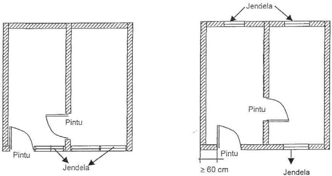
Denah baik, ditinjau dari rencana struktur maupun sistim aliran udara (ventilasi)
