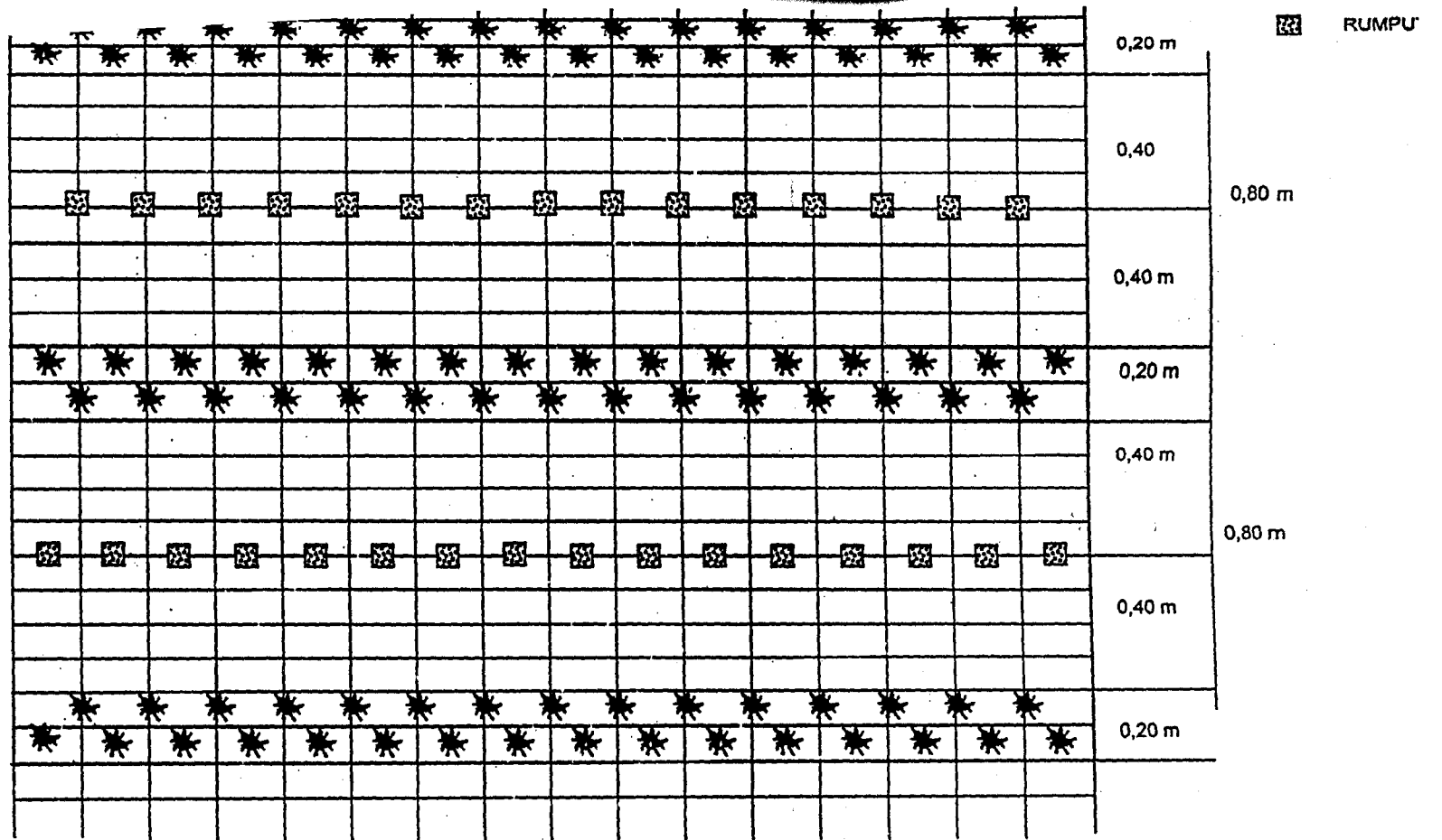
TAMPAK ATAS TATA LETAK PENANAMAN RUMPUT VETIVER PADA LERENG/TEBING 45 DERAJAT
