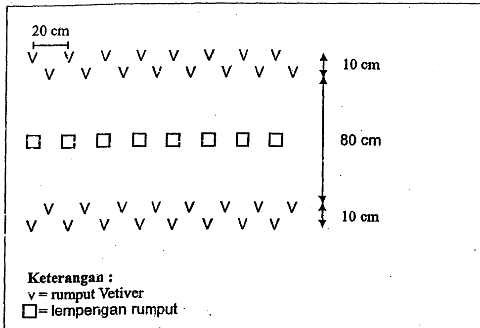
Gambar 7 – Penempatan berjarak Lempengan rumput untuk jarak vertikal setiap setrip Vetiver = 80 cm
