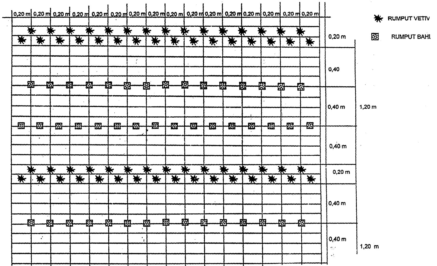
TAMPAK ATAS TATA LETAK PENANAMAN RUMPUT VETIVER PADA LERENG/TEBING 45 DERAJAT
