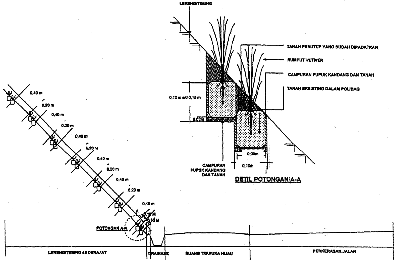
POTONGAN MELINTANG JALAN DAN LERENG/TEBING 45 DERAJAT
