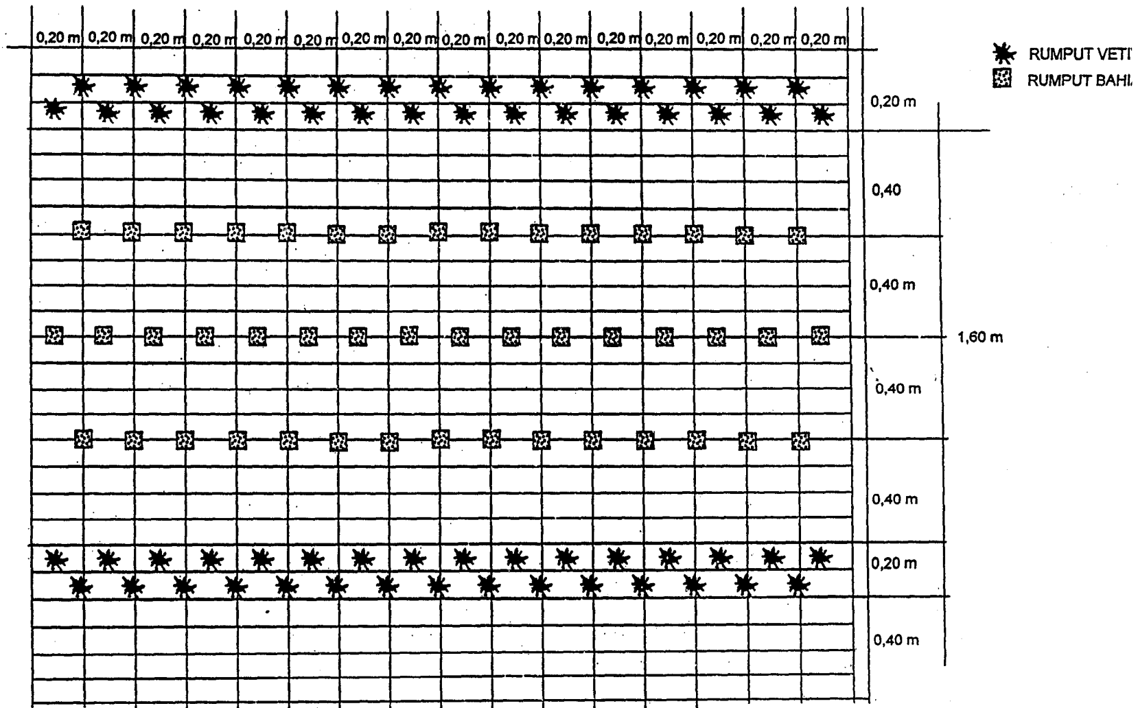
TAMPAK ATAS TATA LETAK PENANAMAN RUMPUT VETIVER PADA LERENG/TEBING 45 DERAJAT
