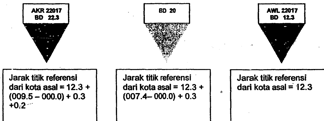
Gambar 13 Ilustrasi pemberian tanda dan informasi titik referensi di badan jalan
