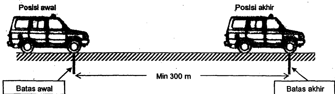
Gambar 10 Posisi kendaraan dalam pelaksanaan kalibrasi IPJ halus
