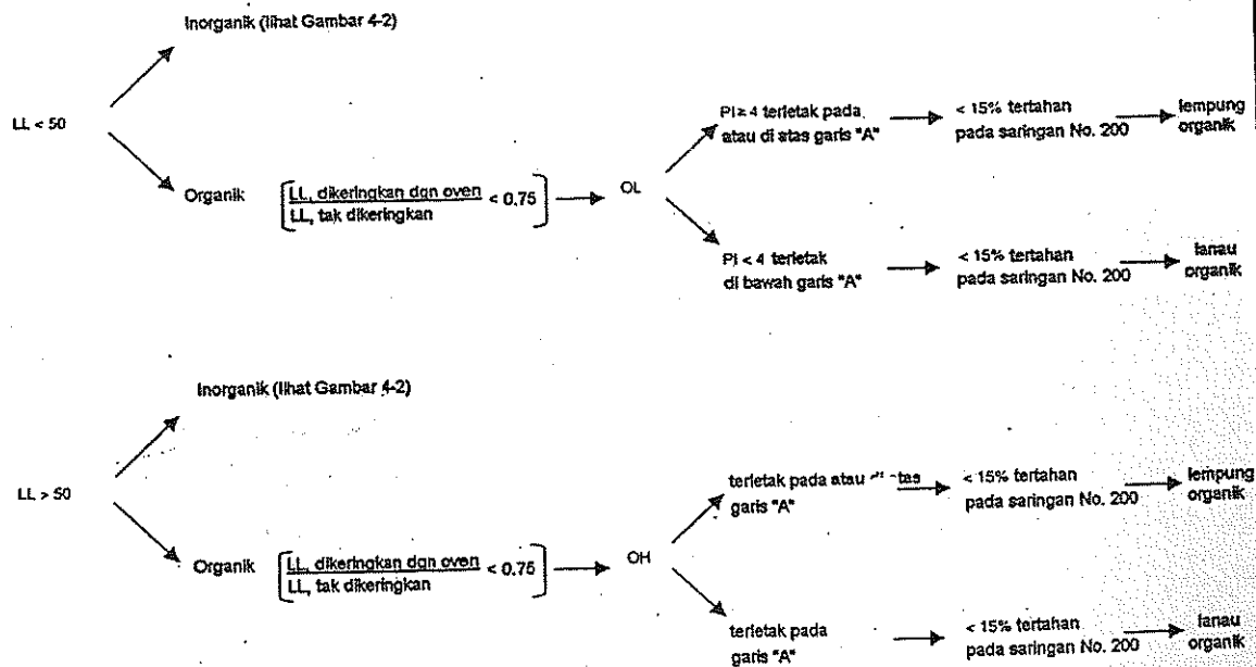
Gambar 4-3 Bagan Alir yang Disederhanakan untuk Mengklasifikasikan Lempung dan Lanau Organik
