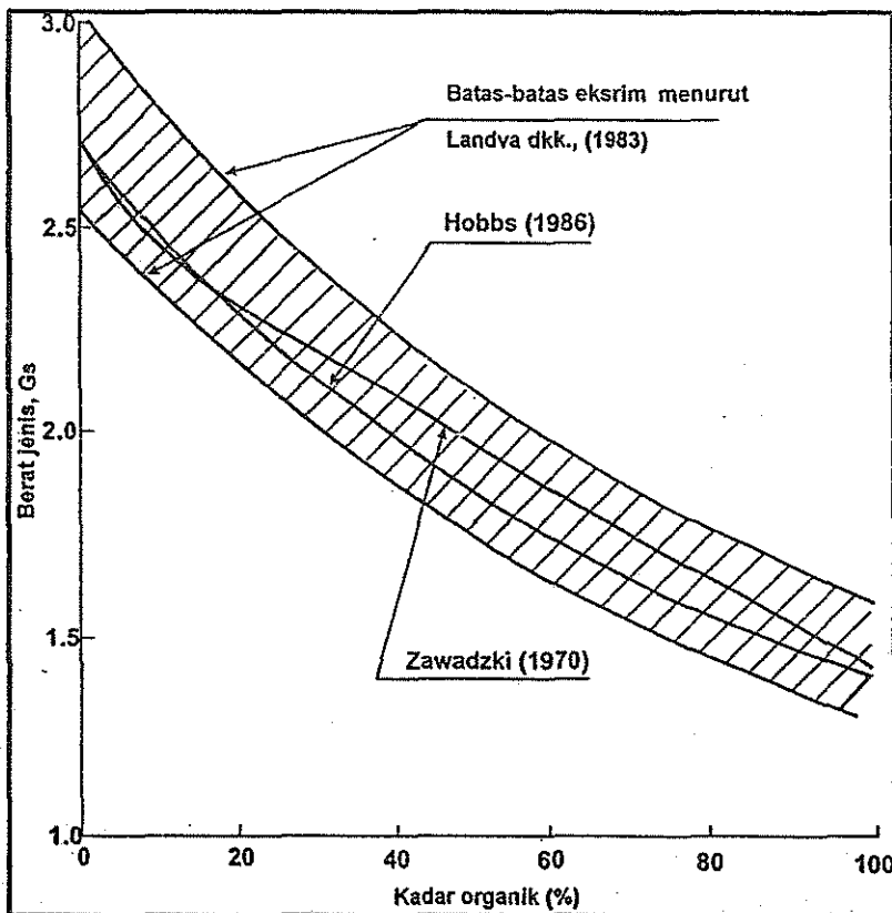
Gambar 4-6 Berat Jenis dan Kadar Organik (Lechowicz dkk., 1996)
