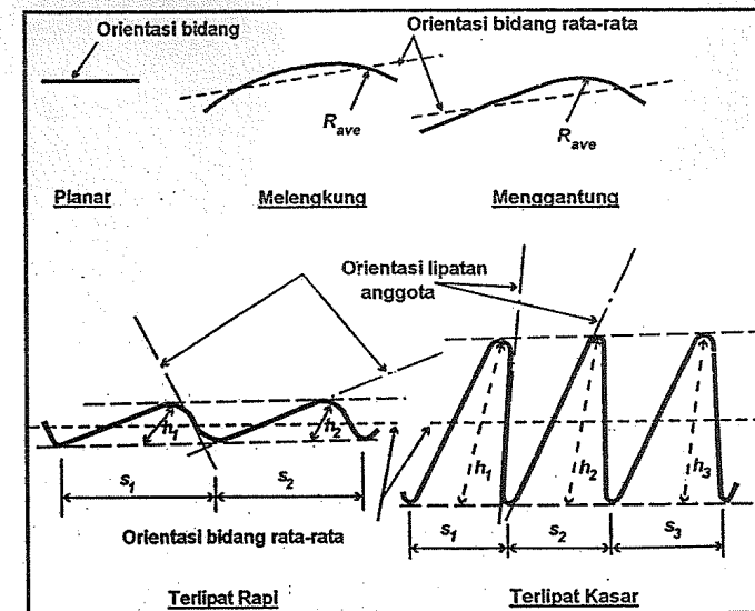
Gambar 6-1 Geometri Permukaan Fitur pada Endapan Bertapis (McGown dan Jarrett 1997a)
