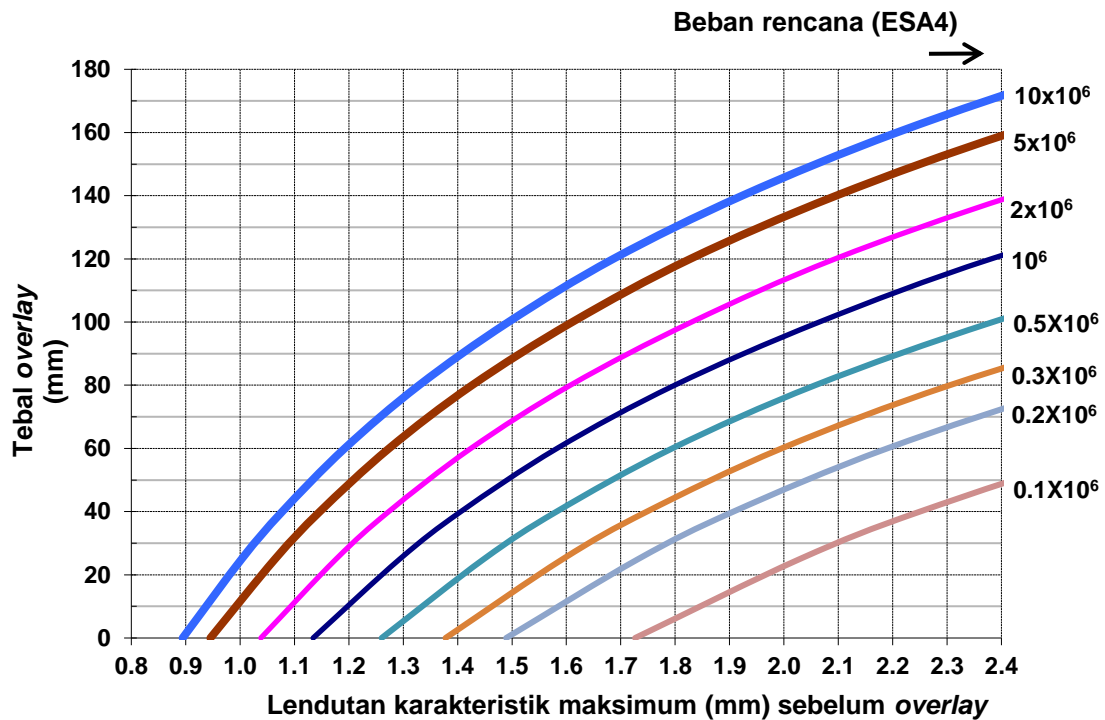
Gambar 6.1. Solusi Overlay Berdasarkan Lentutan Balik Benkelman Beam untuk WMAPT 41°C
