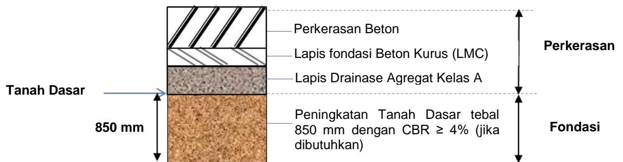
Gambar 1.2. Tipikal Struktur Perkerasan Kaku.
