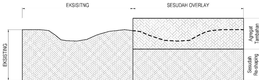
Gambar 8.6. Overlay Perkerasan Tanpa Penutup Aspal
