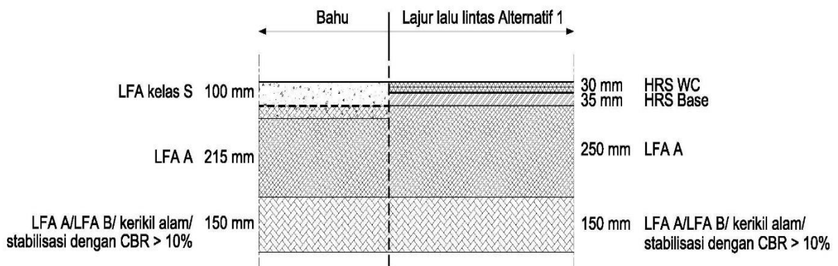
Gambar 10.8. Struktur perkerasan alternatif – 1
