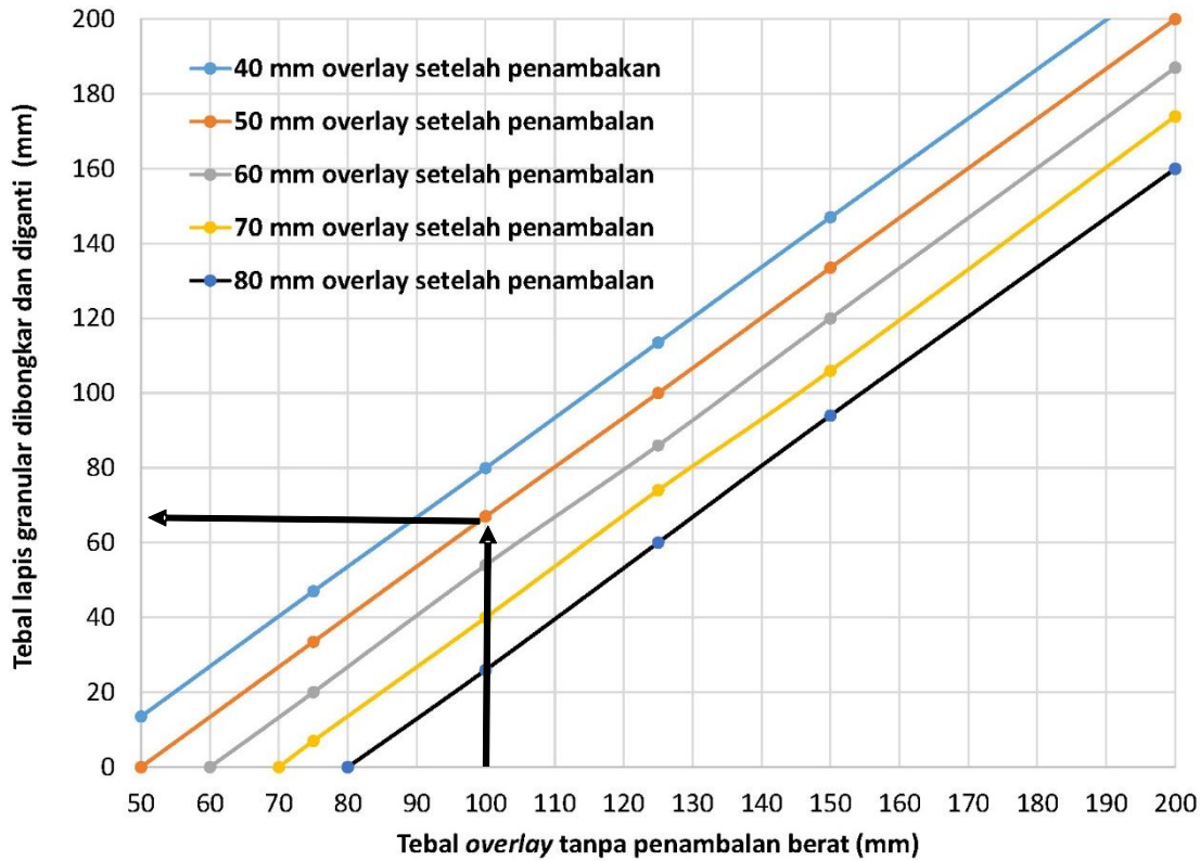
Gambar 10.4. Penentuan tebal pengupasan LPA
