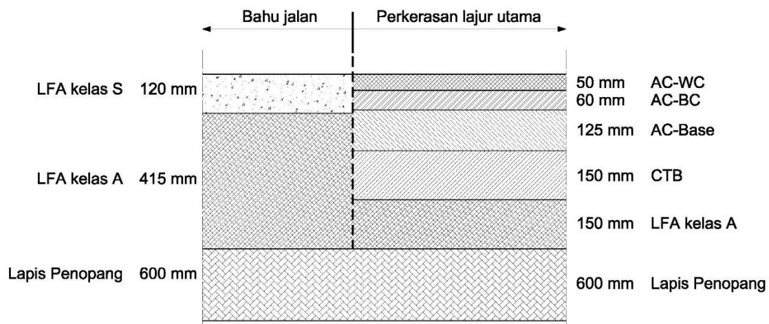
Gambar F.1. Struktur perkerasan alternatif 1
