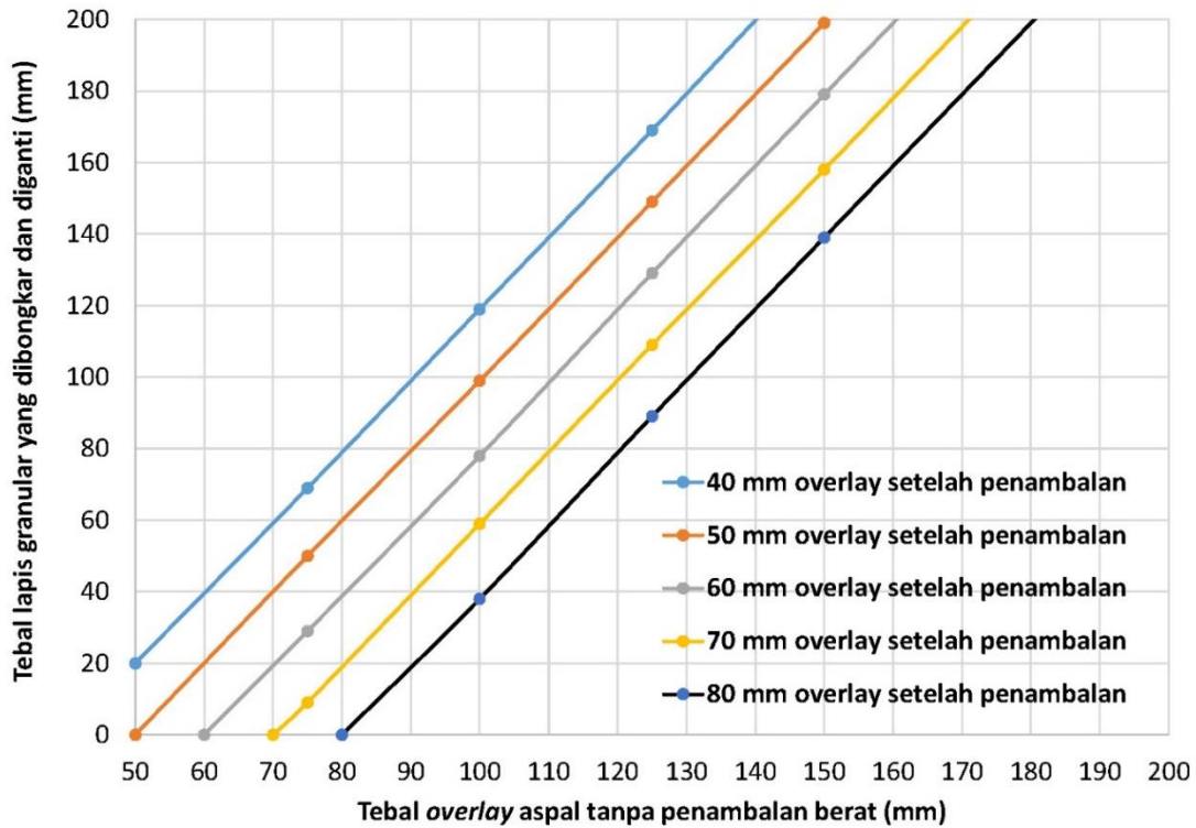
Gambar 7.1. Ketebalan pengupasan lapisan berbutir untuk mencegah deformasi permanen
