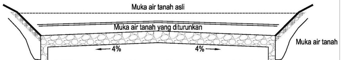
Gambar 5.1 (d) : Lapis penyangkang tidak kedap untuk menurunkan muka air tanah
