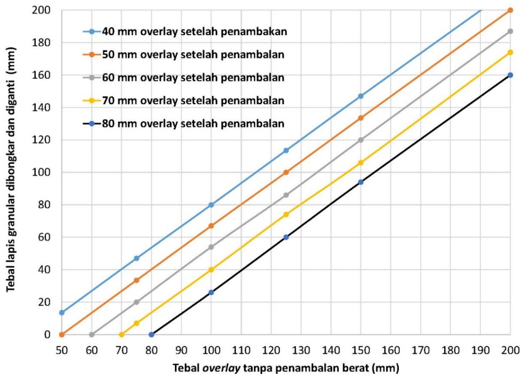
Gambar 7.2. Ketebalan pengupasan lapisan berbutir untuk mencegah fatigue
