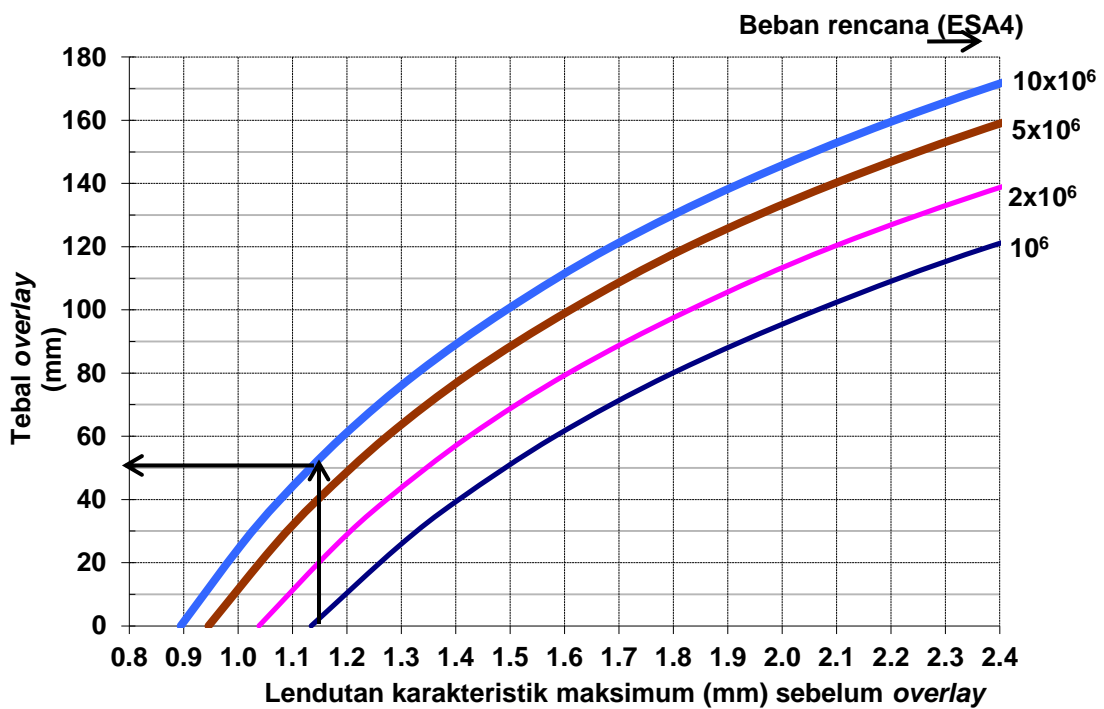
Gambar 10.1. Penentuan tebal overlay berdasarkan D_0
