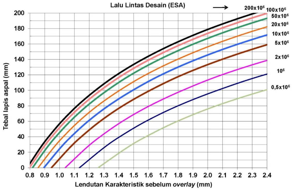
Gambar L.1. Tebal overlay berdasarkan lendutan balik maksimum (Benkelman Beam) (kurva beban > 10x10 6 ESA4 hanya berlaku untuk perencanaan program)
