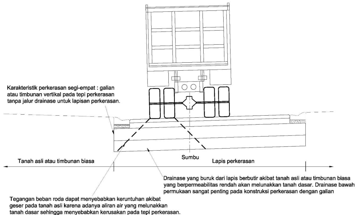
Gambar 8.3. Konstruksi Perkerasan pada Galian Segi Empat (Kasus Tipikal).
