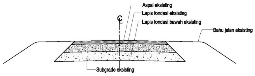
Perkerasan lama (perkerasan yang ada)
