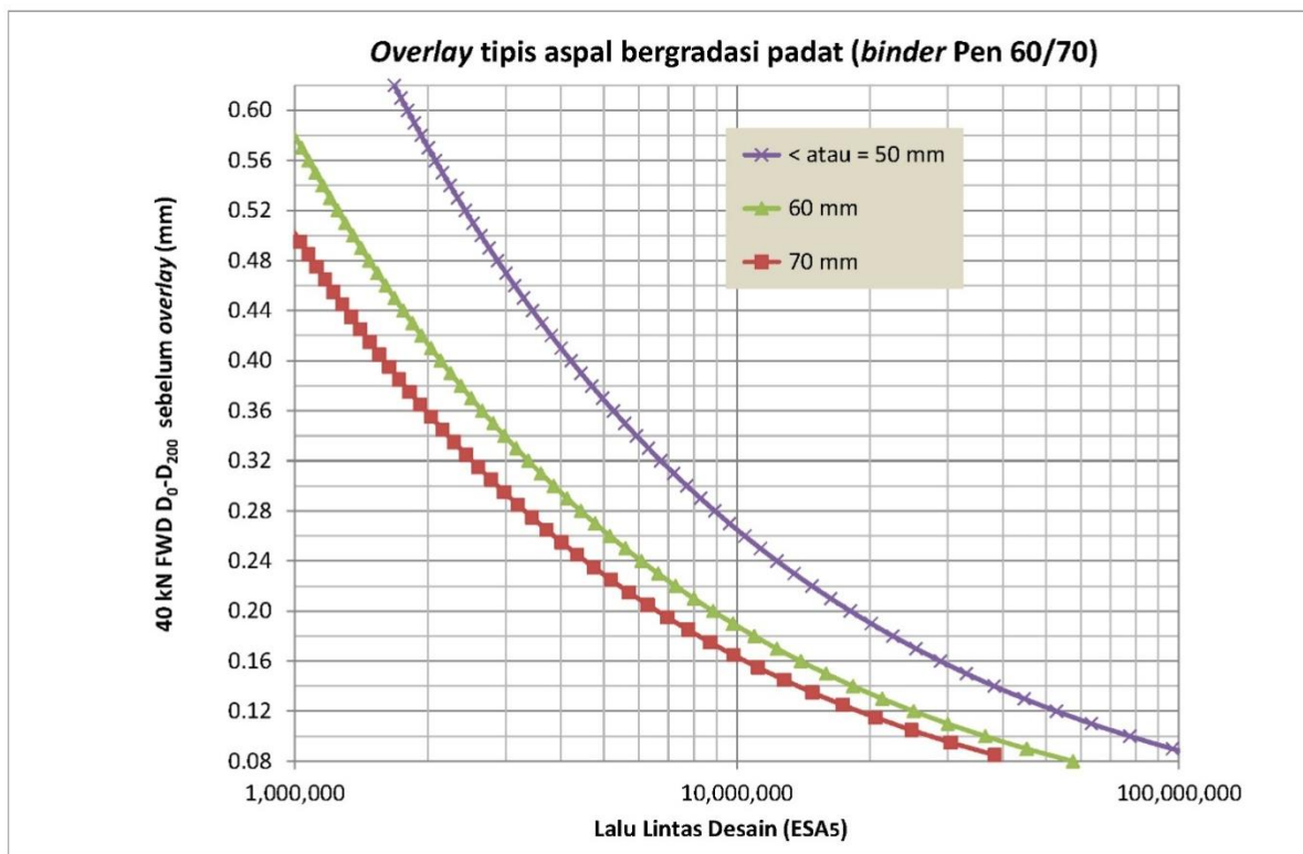
Gambar L.2a. Tebal overlay tipis berdasarkan lengkung lendutan (FWD) (kurva beban > 20x10 6 ESA5 hanya berlaku untuk perencanaan program)
