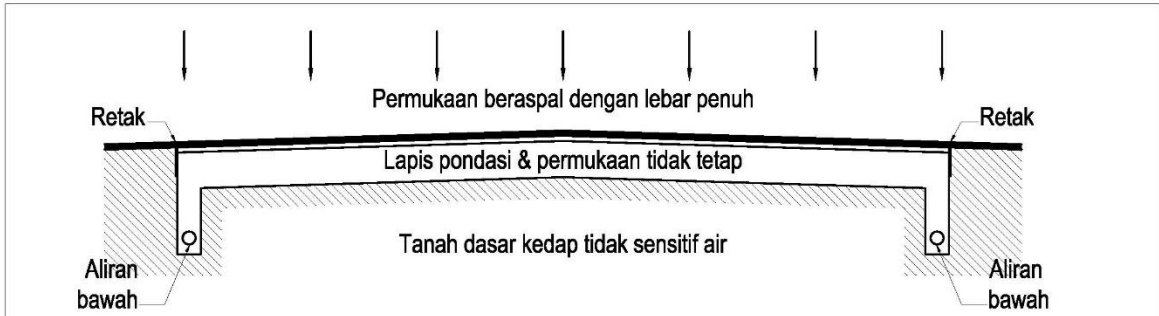
Gambar 5.1 (a) : Infiltrasi permukaan perkerasan dengan tanah dasar segiempat
