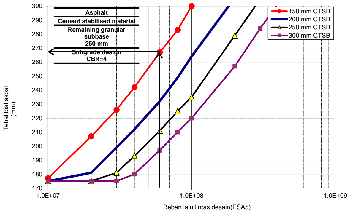
Gambar 10.5. Penentuan tebal lapisan CTSB dan aspal
