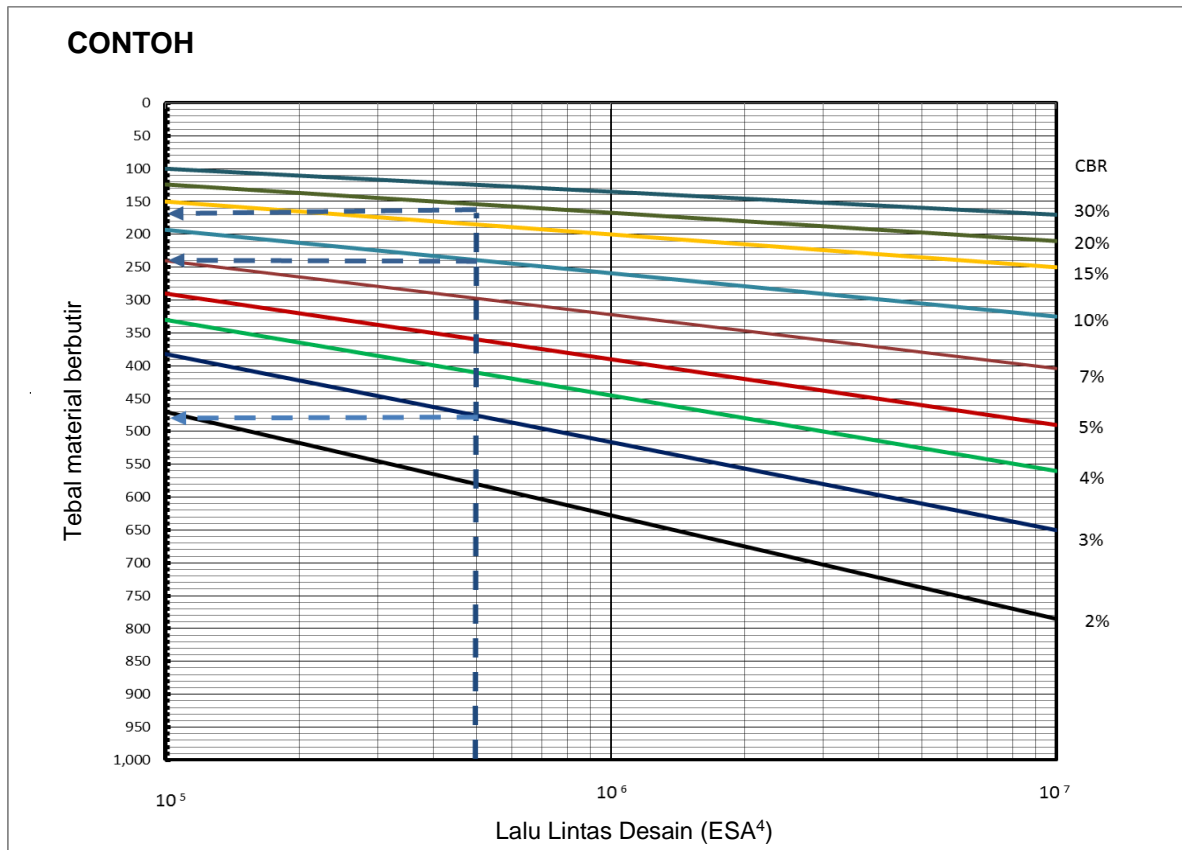
Gambar E.1. Contoh penggunaan desain 7 untuk Perkerasan Tanpa Penutup Aspal
