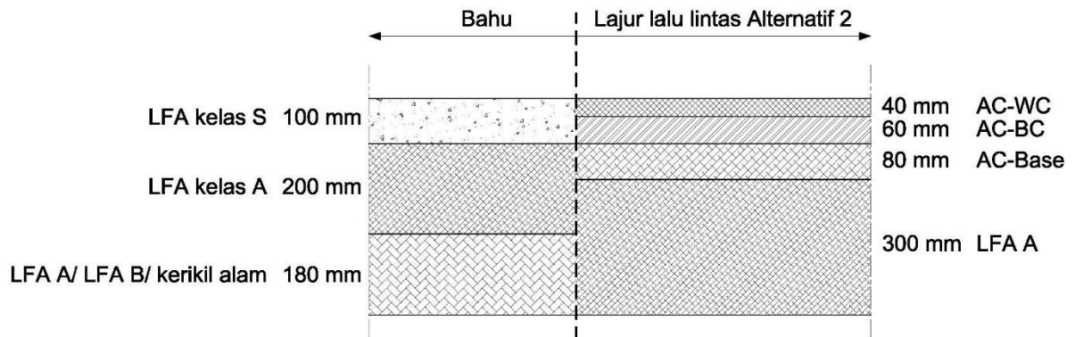
Gambar 10.9. Struktur perkerasan alternatif – 2
