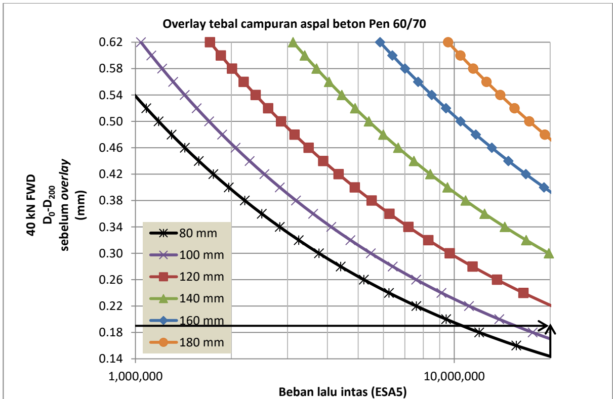
Gambar 10.2. Penetapan tebal overlay (tipis)
