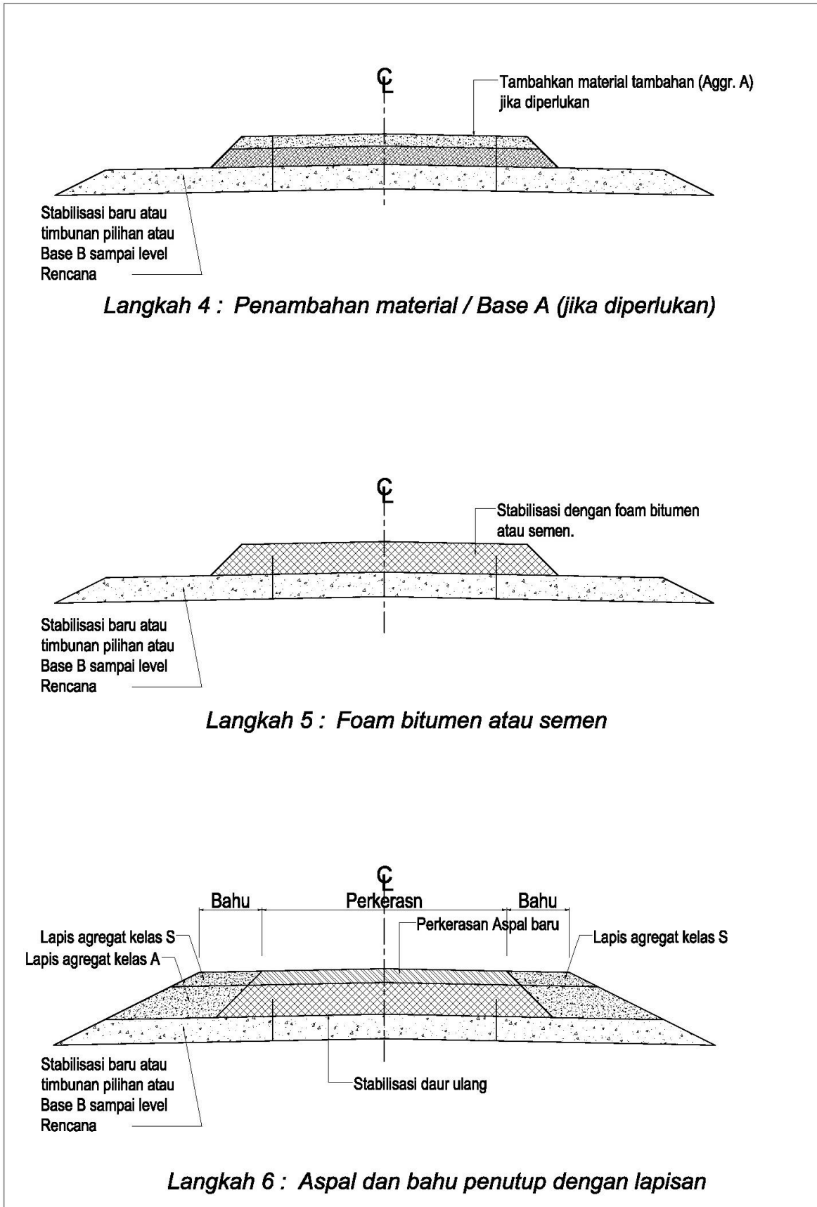
Gambar 9.1. Urutan Pelaksanaan Daur Ulang dengan Pelebaran
